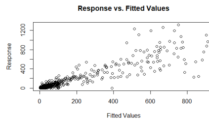
(d) Response against Fitted values
