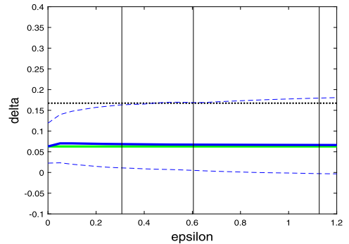
(d) n_X = 20
