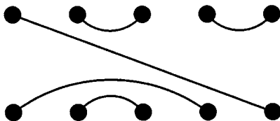
FIG. 1. An r -digram ( r = 5 ).
