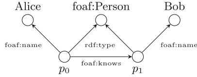
Fig. 1. RDF Dataset
