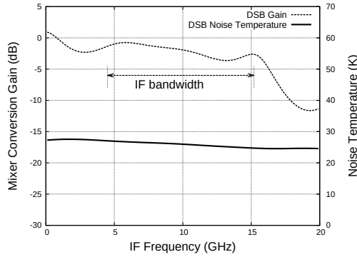
(d) IF response for direct-mixers (SOI substrate)
