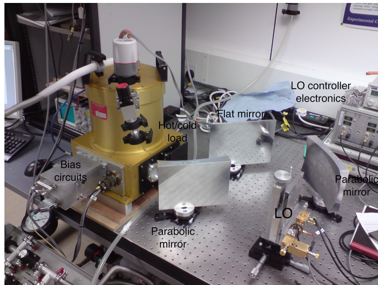
(a) Actual experimental setup
