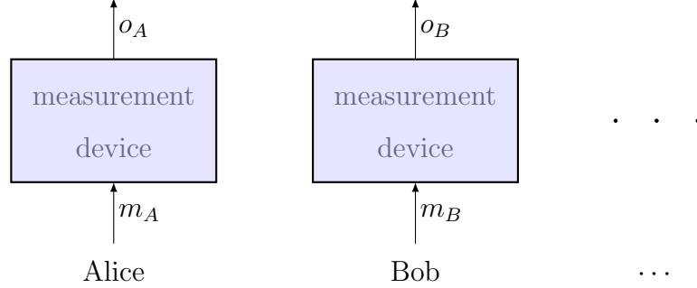
Figure 4.1: A Bell scenario.
