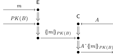
(d) A Fake subpath for A, B \in \mathcal{T}_{names}^{reg} .
