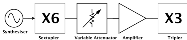
Fig. 3 LO chain block diagram.
